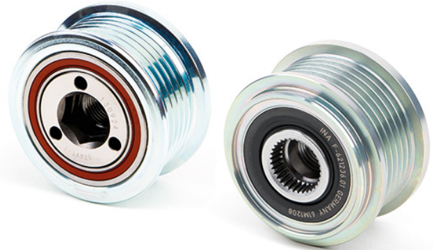
Bild: Optische Unterschiede des Generatorfreilaufs 535 0303 10
