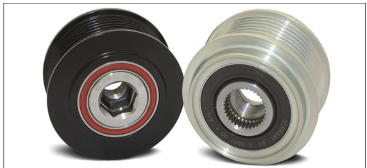
Bild 2: Generatorenfreilauf 535 0229 10
