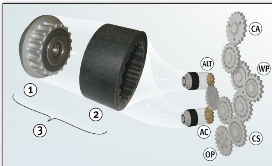
Bild 1: Generatorfreilauf mit flexibler Kupplungsmuffe und Stirnradtrieb
